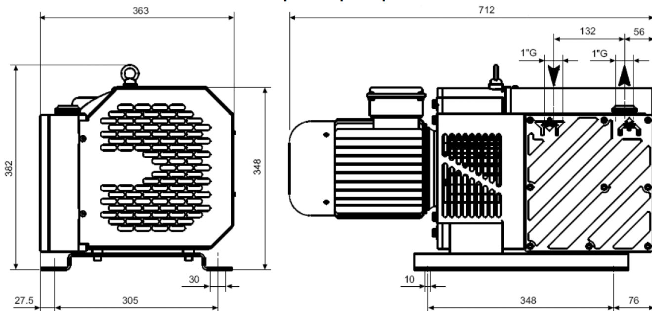
Габаритные размеры.
