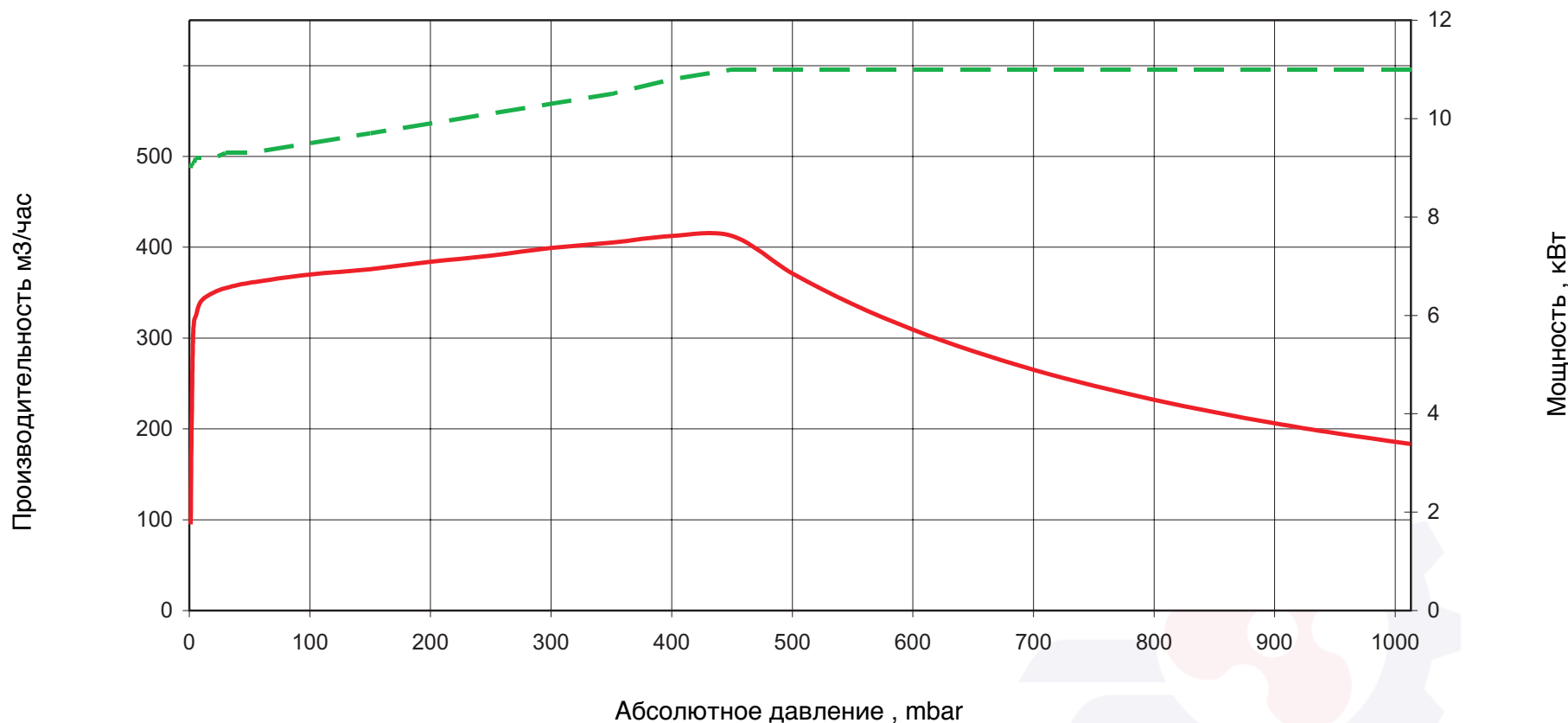
График работы насоса UV8
