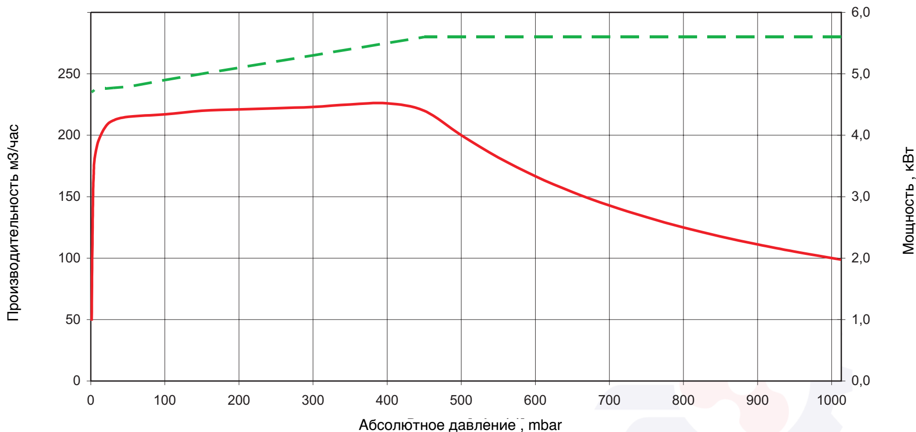
График работы насоса UV4
